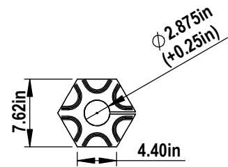
2 8" HELIX N.T.S.
