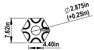
2 8" HELIX N.T.S.
