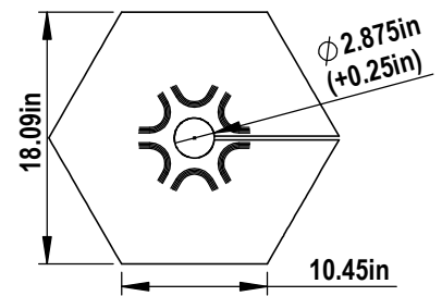
2 19" HELIX N.T.S.
