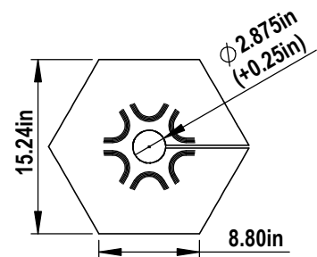
2 16" HELIX N.T.S.
